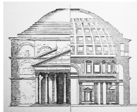
Schnitt durch das römische Pantheon, James Ferguson, A History of Architecture in All Countries, London 1893
