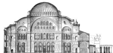
Längsschnitt durch die Hagia Sophia
